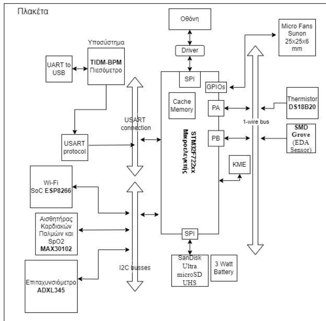
Εικόνα. 1: Αρχιτεκτονική Υλικού
